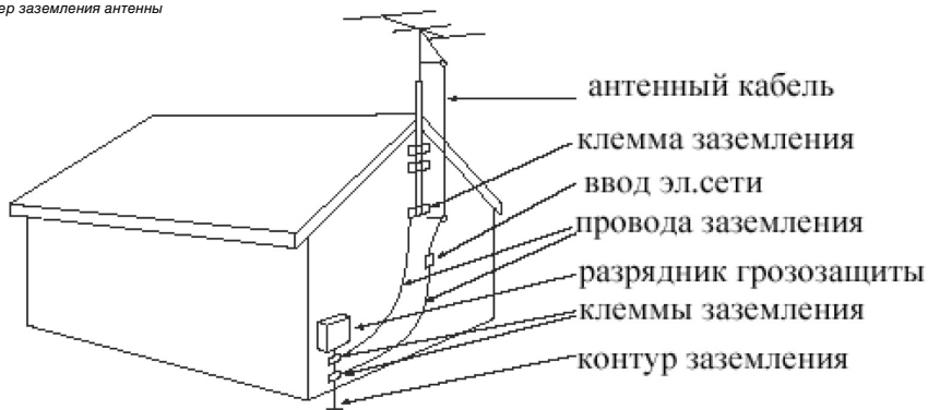
Рис. А. Пример заземления антенны
